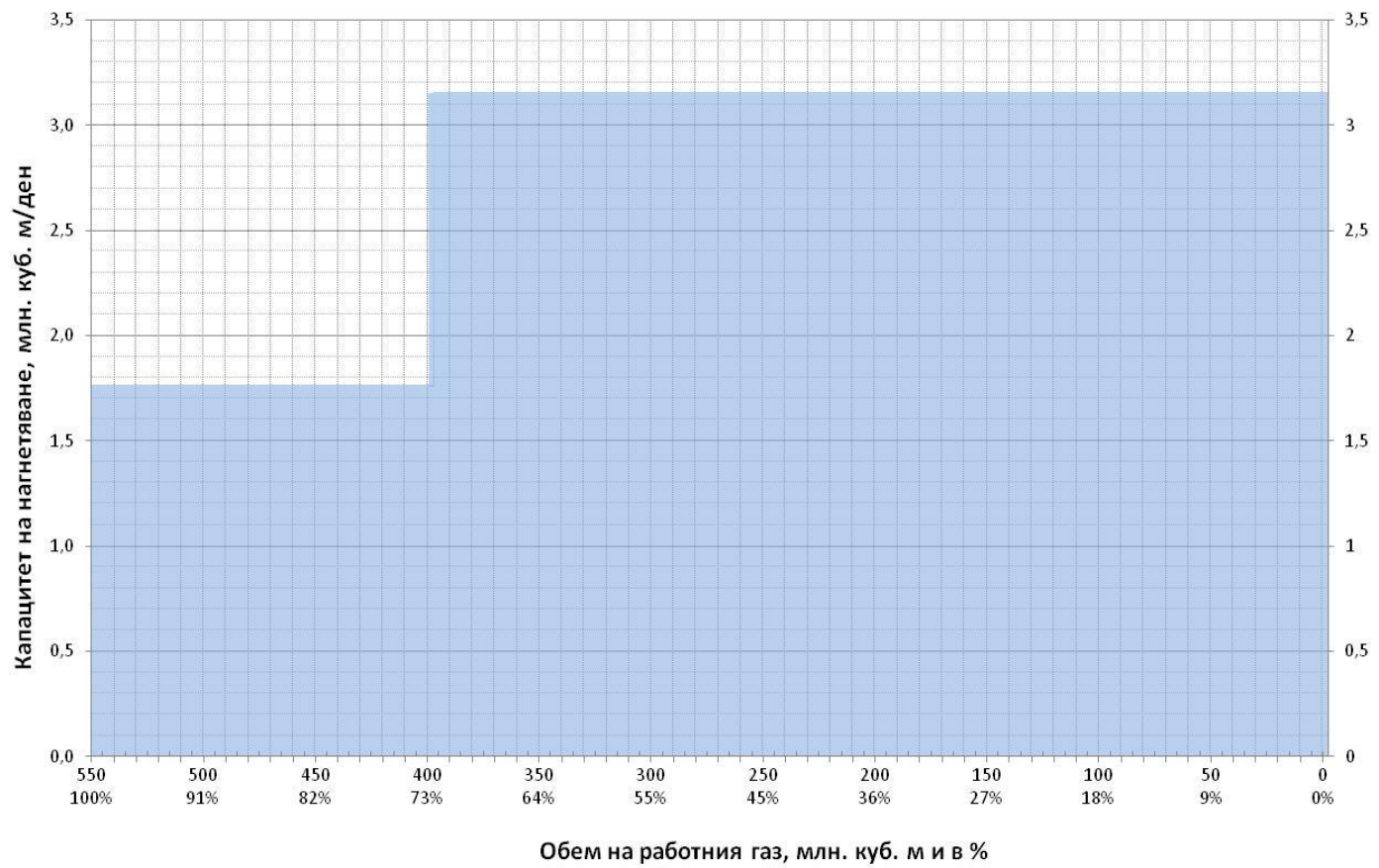
Крива на капацитета на нагнетяване на ПГХ Чирен за газова година 2014-2015, млн. куб. м
